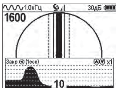
Рис.А.3 КЗ-однофазное
