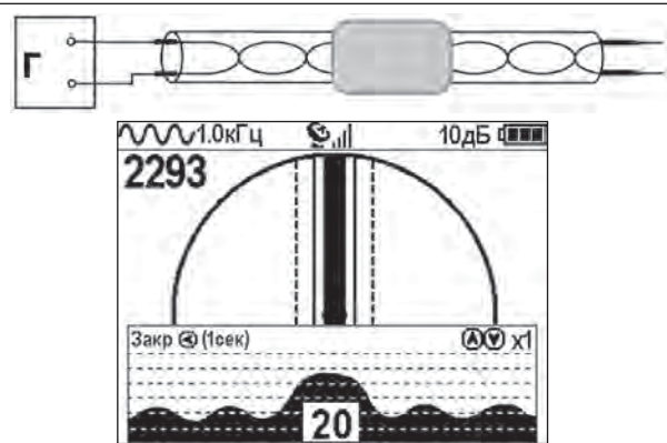
Рис.А.2 Муфта
