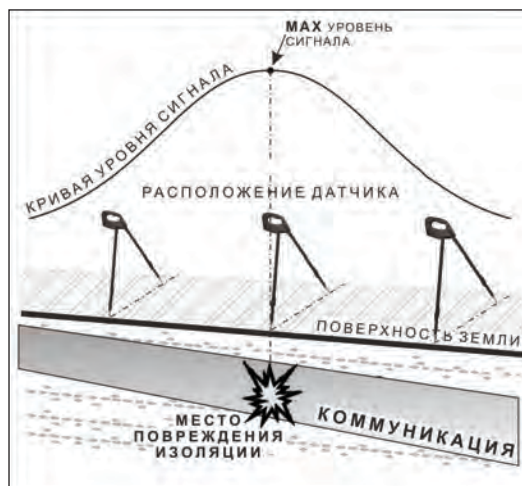
применение датчика контроля изоляции (ДКИ) методом тах
